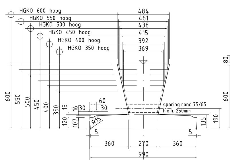
Doorsnede HGKO-ligger SCHAAL 1:20
