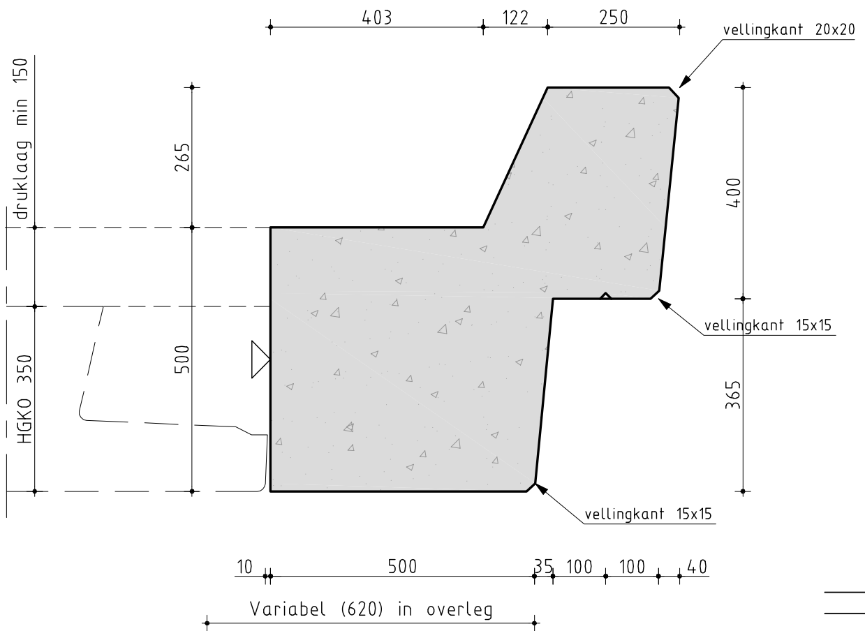
Doorsnede HGR-500-ligger
