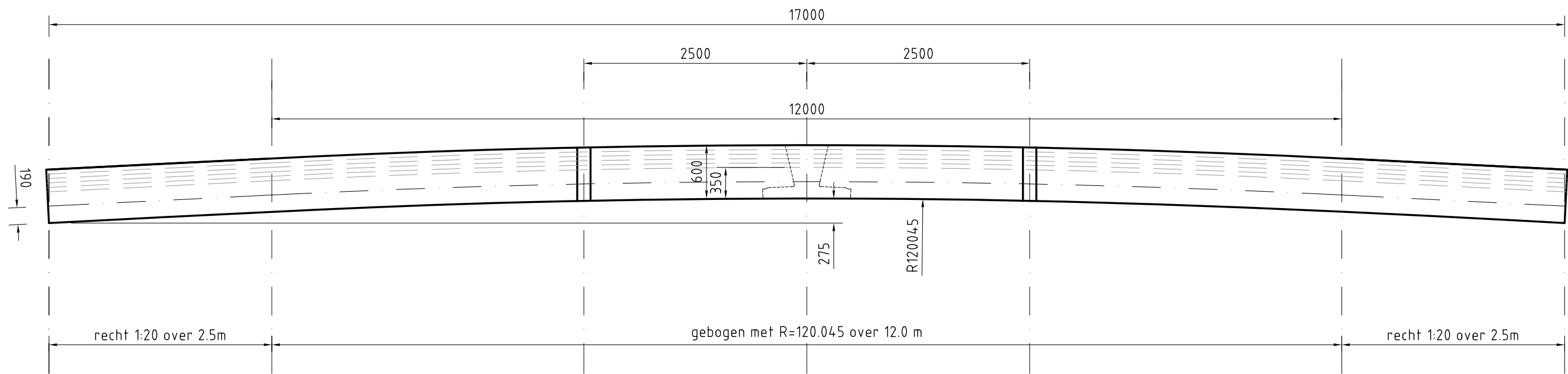
ZIJAANZICHT HGKO
