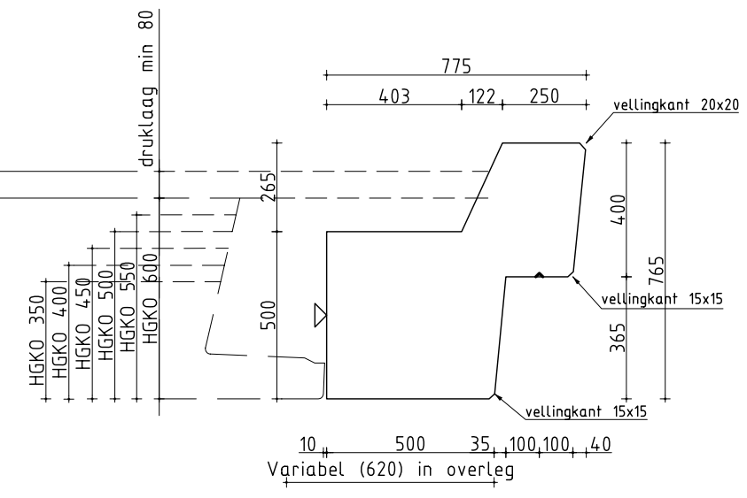
Doorsnede HGR-ligger SCHAAL 1:20
