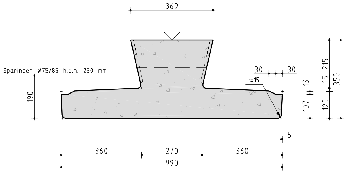
Doorsnede HGK0-350-ligger
