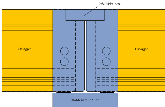
Oplegdetail tussensteunpunt met buigslappevoeg (statisch onbepaald)
