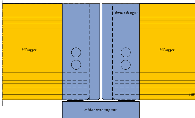
Oplegdetail tussensteunpunt met voeg (statisch bepaald)
