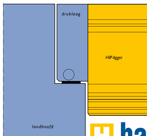
Oplegdetail landhoofd met tandoplegging (statisch bepaald)
