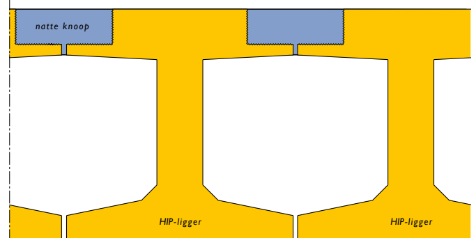
Dwarsdoorsnede HIP-ligger
