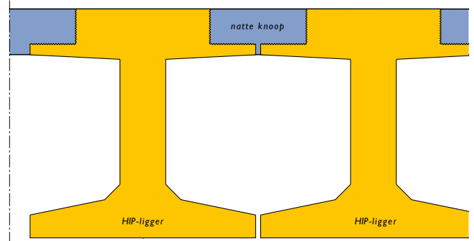
Dwarsdoorsnede HIP-ligger
