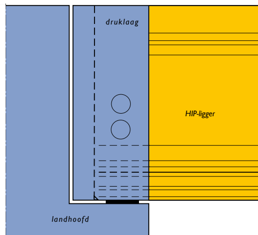
Oplegdetail landhoofd (statisch bepaald)
