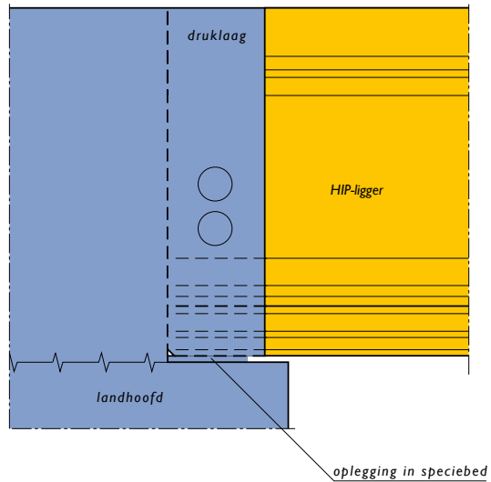
Oplegdetail landhoofd (statisch bepaald)
